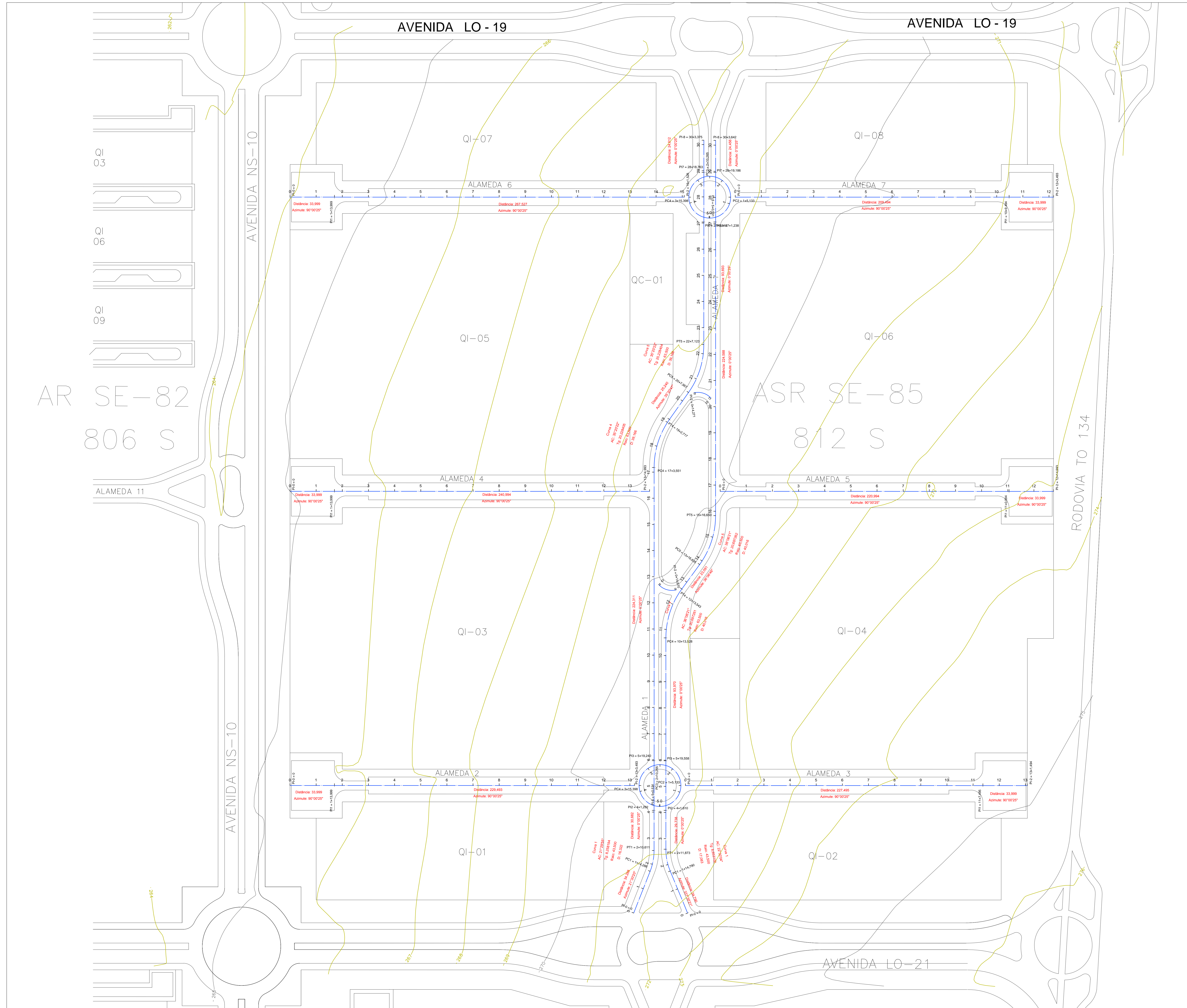
Planta de Terraplanagem Escala: 1 / 1.000
