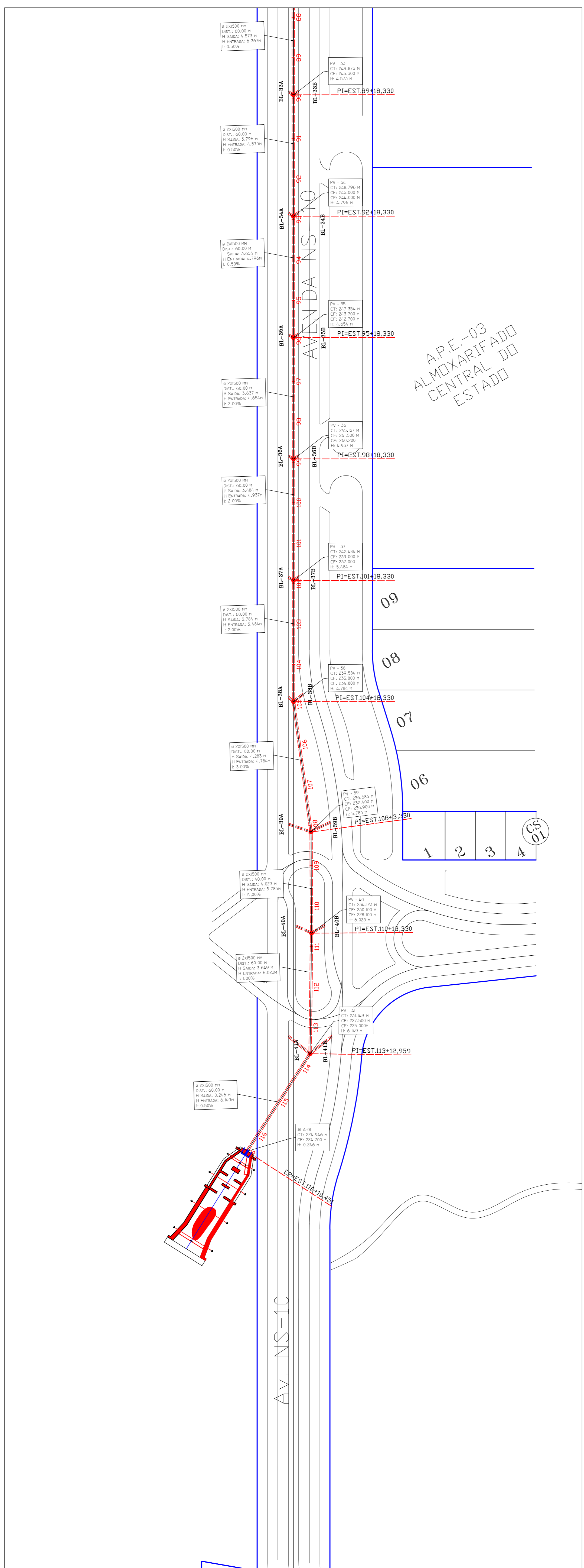
Planta de Drenagem - 4 Escala: 1 / 1.000
