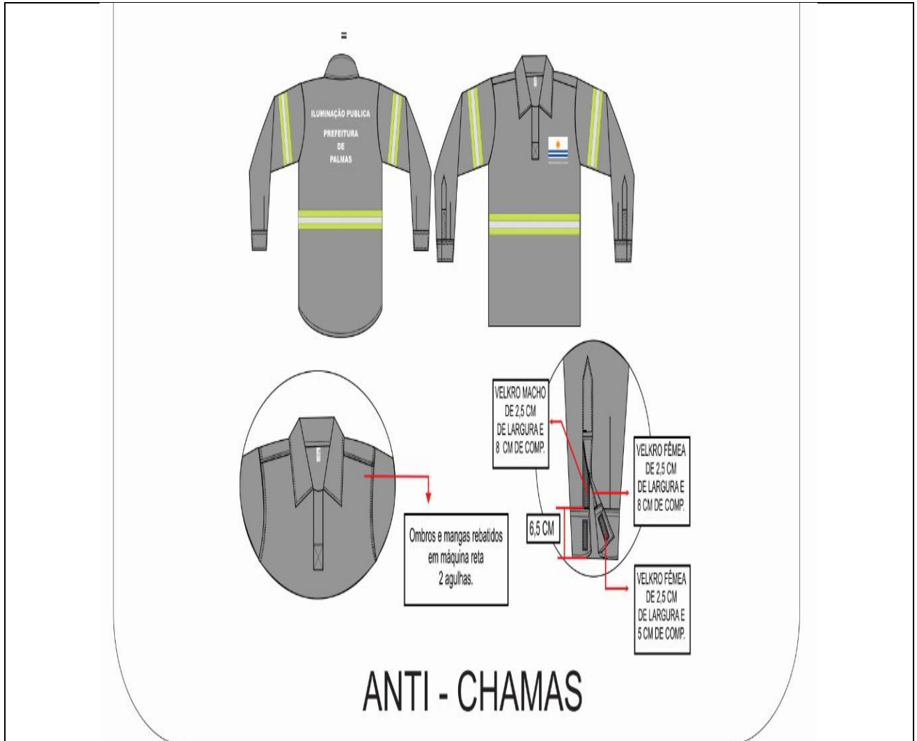
Figura 02: Jaleco profissional para eletricista com Faixa Refletiva, antichamas.
