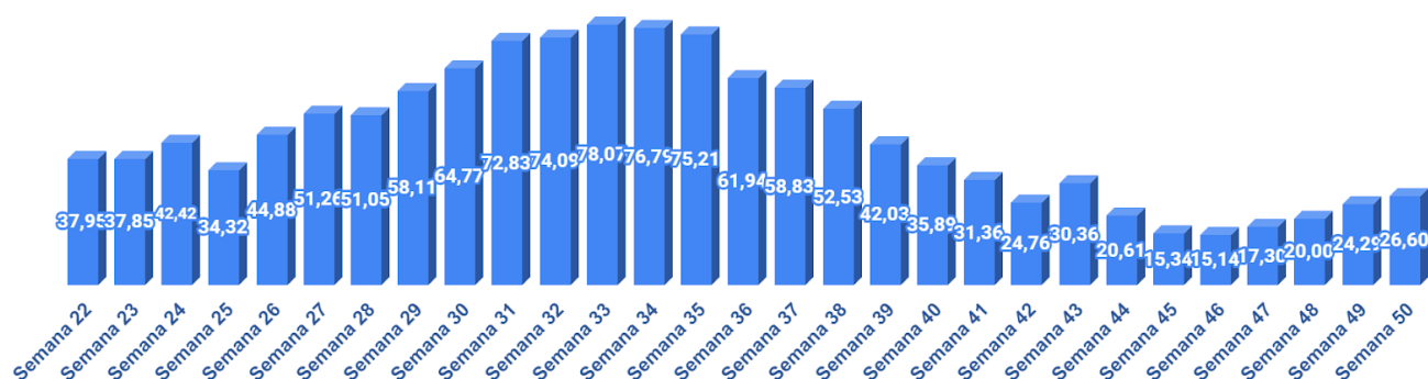
Gráfico 7. Média da taxa de ocupação total de leitos hospitalares localizados em Palmas-TO por semana epidemiológica, 2020.
