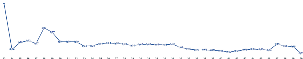
Gráfico 5. Média do R_0^* por semana epidemiológica em Palmas-TO, 2020.
