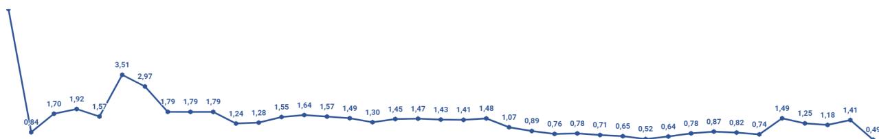
Gráfico 5. Média do R_0^* por semana epidemiológica em Palmas-TO, 2020.
